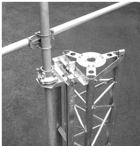
タワー頂部
