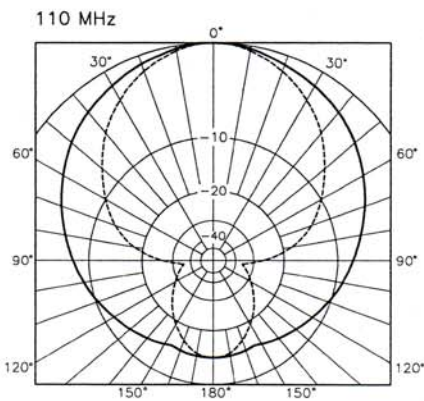
CLP5130-1x 50~500MHz
