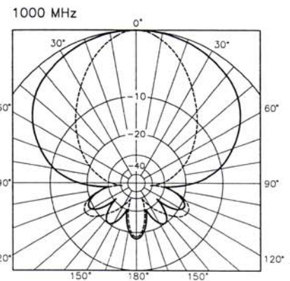
CLP3100 30~1000MHz
