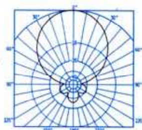
水平面パターン /18m高
